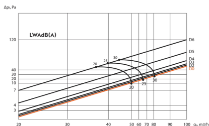
LINEO 600, 20 mm slot (odvod vzduchu)
