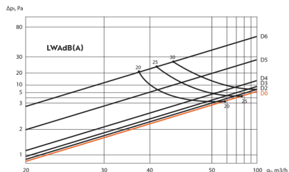
LINEO 600, 20 mm slot (přívod vzduchu)
